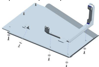
29-T020202 kryt motoru pro vozy s montážní sadou hidden
