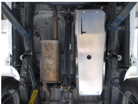
29-T010102FFB kryt nádrže
